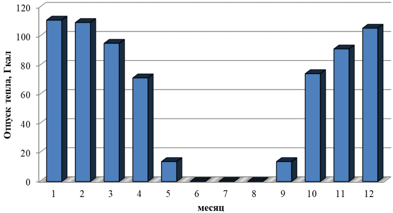
Рисунок 1.2 – Оптимальный температурный график отпуски тепловой энергии для котельной школы
