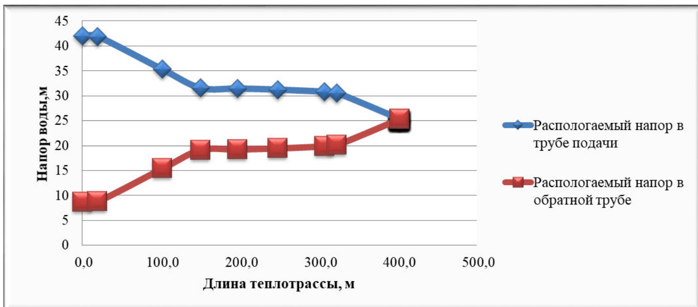
Рисунок 2.6 – Пьезометрический график тепловой сети котельной клуба по магистральному выводу
