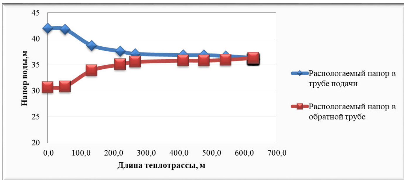
Рисунок 2.3 – Пьезометрический график тепловой сети котельной школы по магистральному выводу
