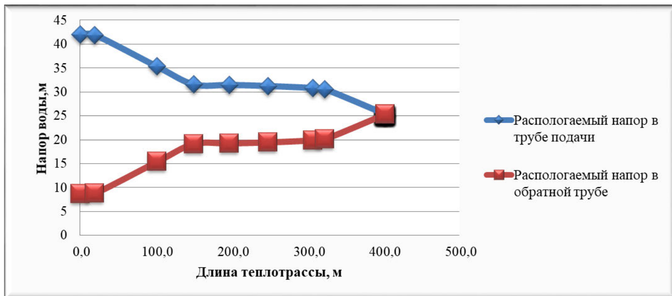
Рисунок 2.4 – Пьезометрический график тепловой сети котельной клуба по магистральному выводу
