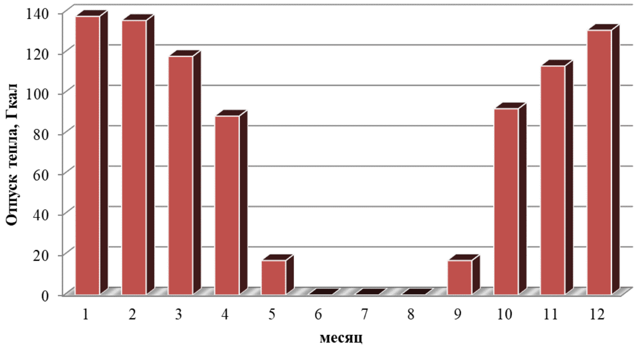
Рисунок 1.3 – Оптимальный температурный график отпуски тепловой энергии для котельной клуба
