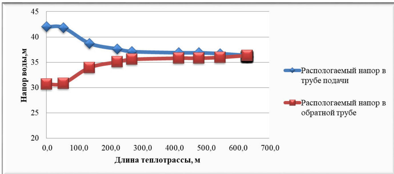
Рисунок 2.5 – Пьезометрический график тепловой сети котельной школы по магистральному выводу
